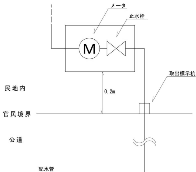
図－３ メータ標準設置図
